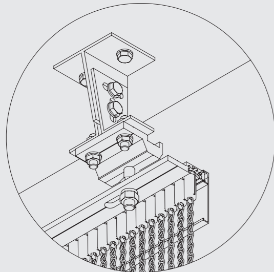
Concrete fixing Fijación a hormigón
